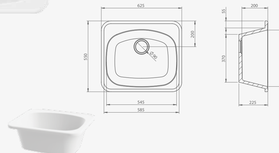
JEDNODJELNI ugradbeni built-in nadgradbeni semi built-in
