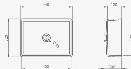
CLARION MINI ugradbeni built-in
