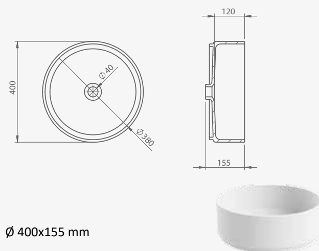
ARENA ugradbeni built-in ugradnja na pult installation on a table top
